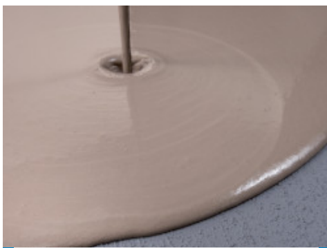
Aplicação de barramento autonivelante sobre Eco Prim Grip Plus seco e aplicado sobre pavimento velho
