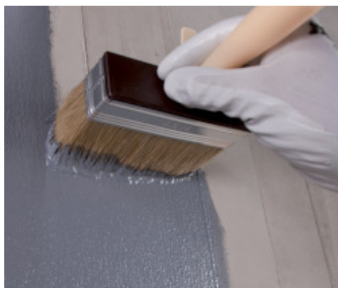
Aplicação de Eco Prim Grip Plus com pincel sobre suporte em betão
