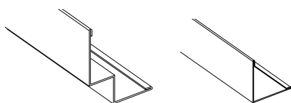
Cantoneira em L e Duplo L (00PL e 0PLL)
